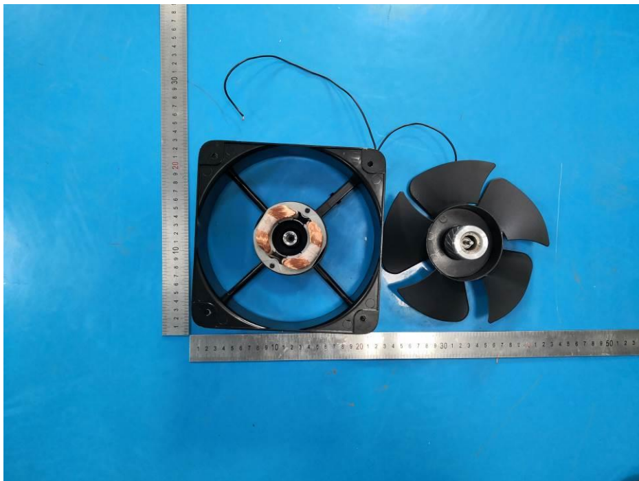
内部结构
