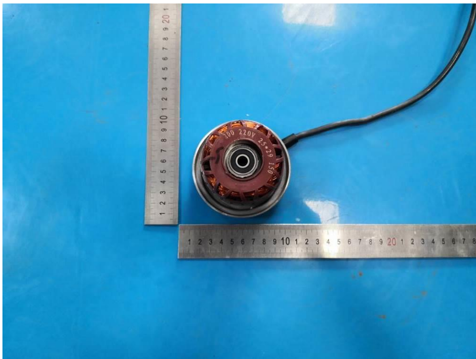
定子
