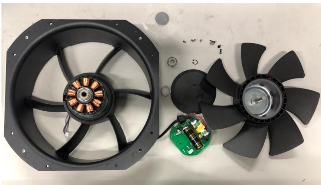
2#样品散件
