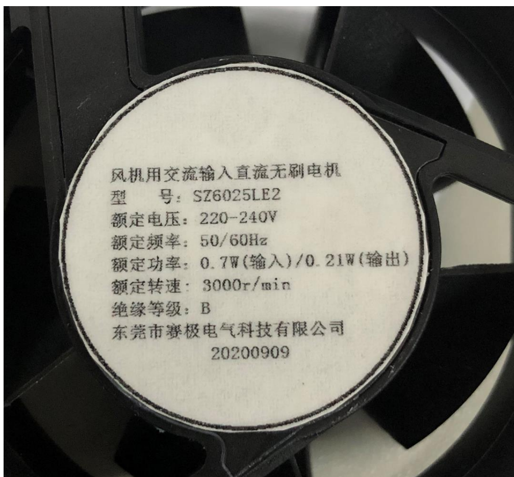
1#样品铭牌
