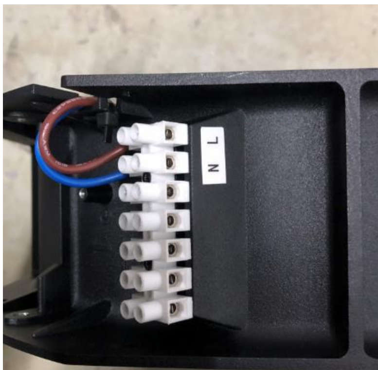
2#样品引出线引出端
