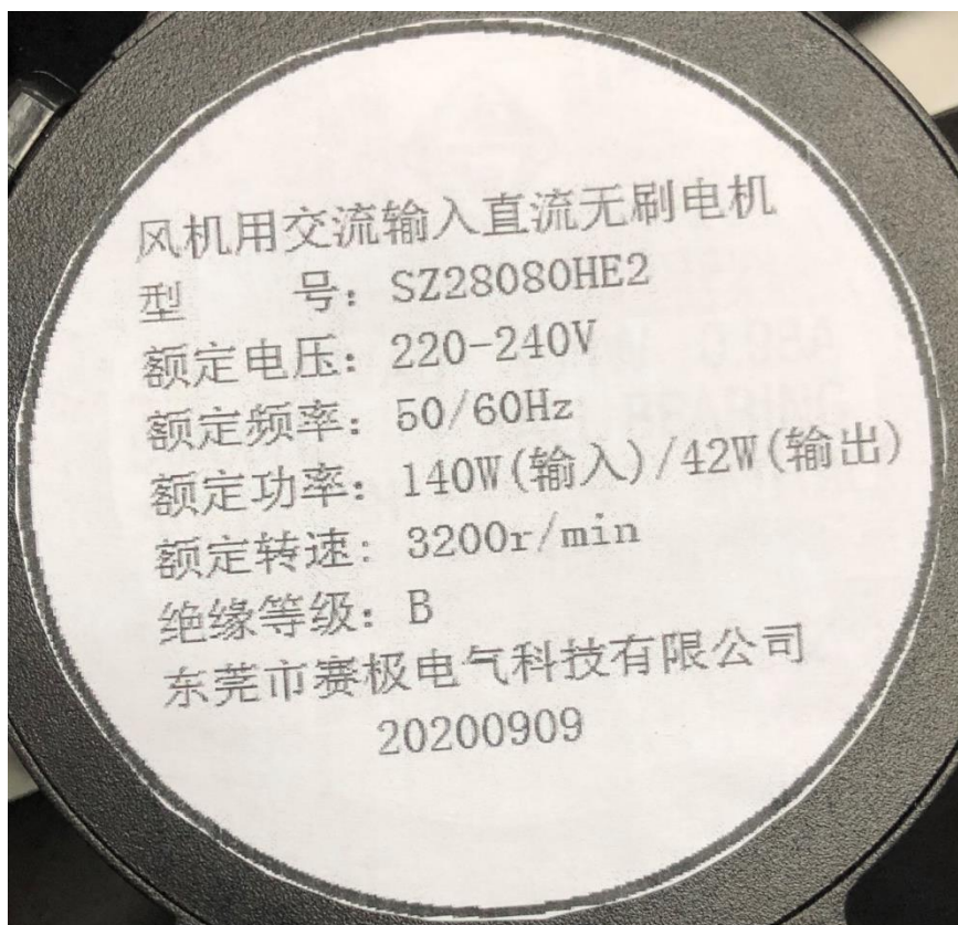
2#样品铭牌
