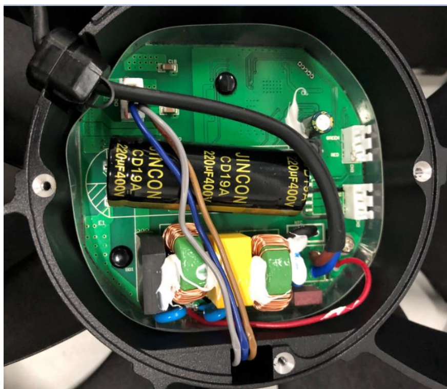
2#样品电子线路板
